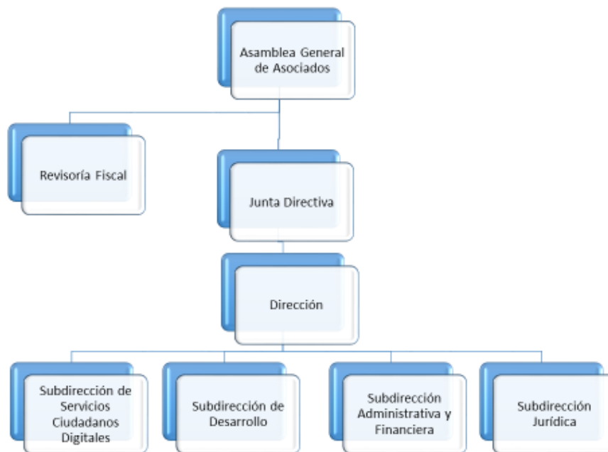
Ilustración 4. Organigrama AND
